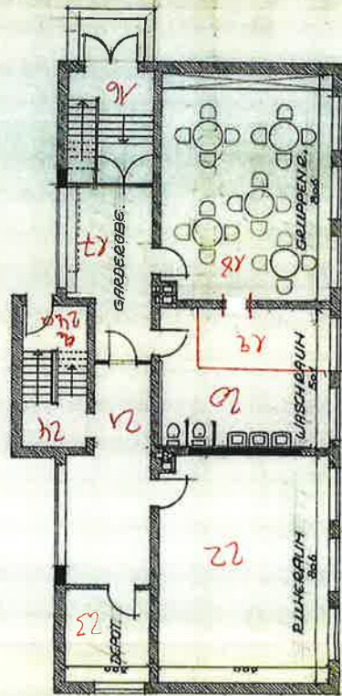
ERDGESCHOSS
