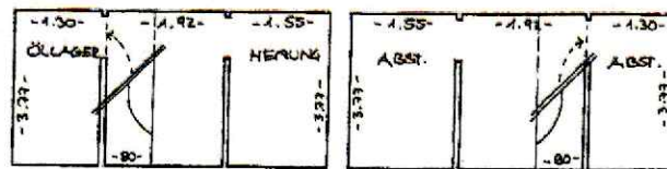
GRUNDRISS KG
