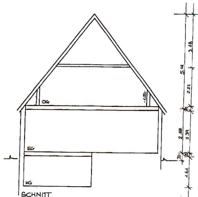
SCHNITT
